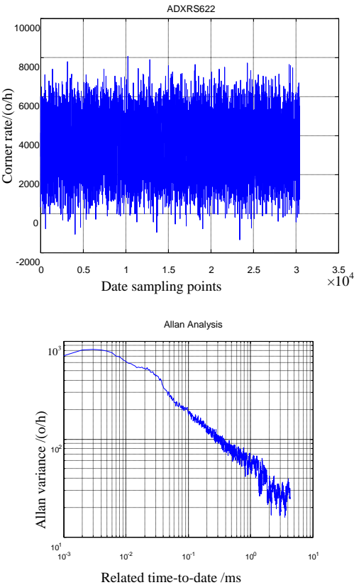
图3 Allan 方差分析结果
