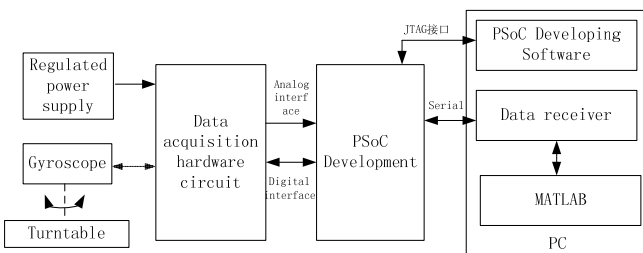
图 1 PSoC 陀螺仪数据采集系统结构
