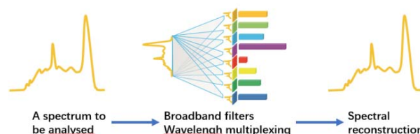
图7 微型量子点光谱仪工作原理
