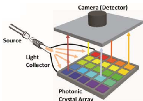
图6 光子晶体微型光谱仪工作原理
