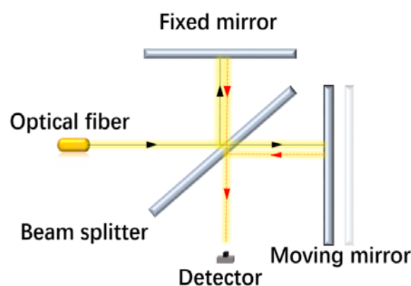
图3 迈克尔逊干涉仪工作原理
