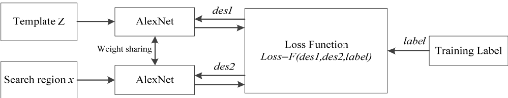
图1 Siamese 全卷积跟踪网络 示, 该网络包含基本网络、侧边输出模块以及融合模块。
