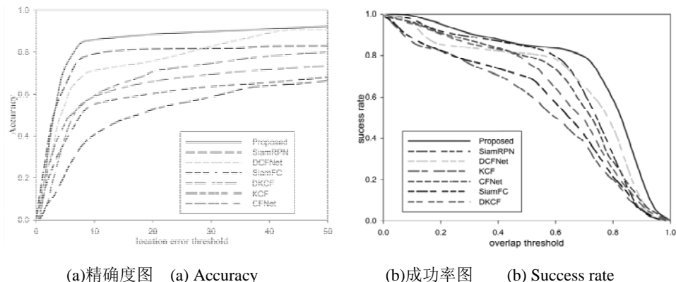
图 5 不同跟踪算法的跟踪性能对比 Fig.5 Comparison of tracking performance for different tracking algorithms
